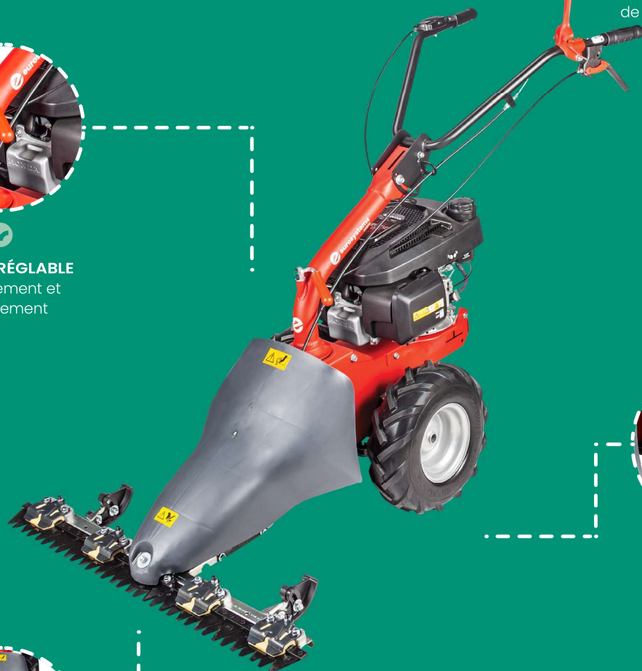
ROUES MOTRICES anti-crevaison 13x5.00-6"
